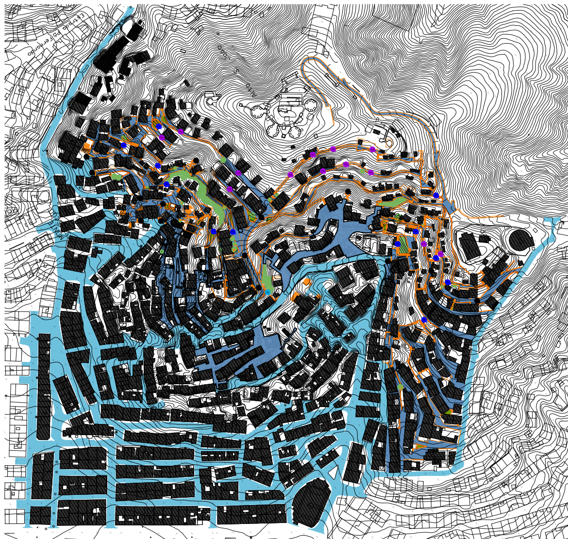
01. ALTO DE BOMBA PLANTA GERAL DE INTERVENÇÃO
